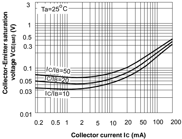
VCE(sat)-IC
